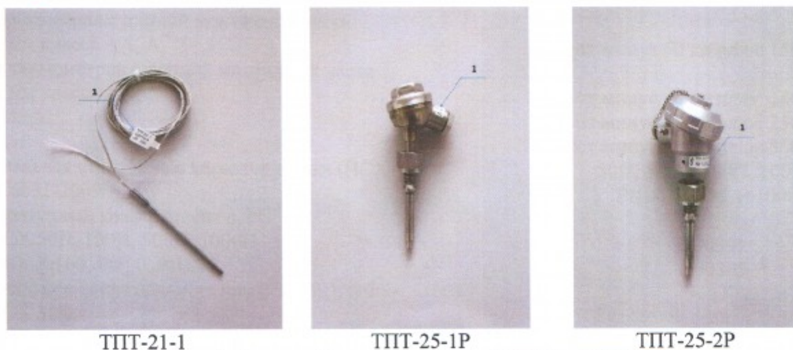
Рисунок 4 – Внешний вид термометров ТПТ-21, ТПТ-25Р (1 – место нанесения маркировки)
